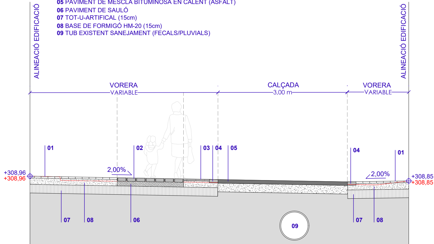
SECCIÓ 2 - SECCIÓ CONSTRUCTIVA E1:50
