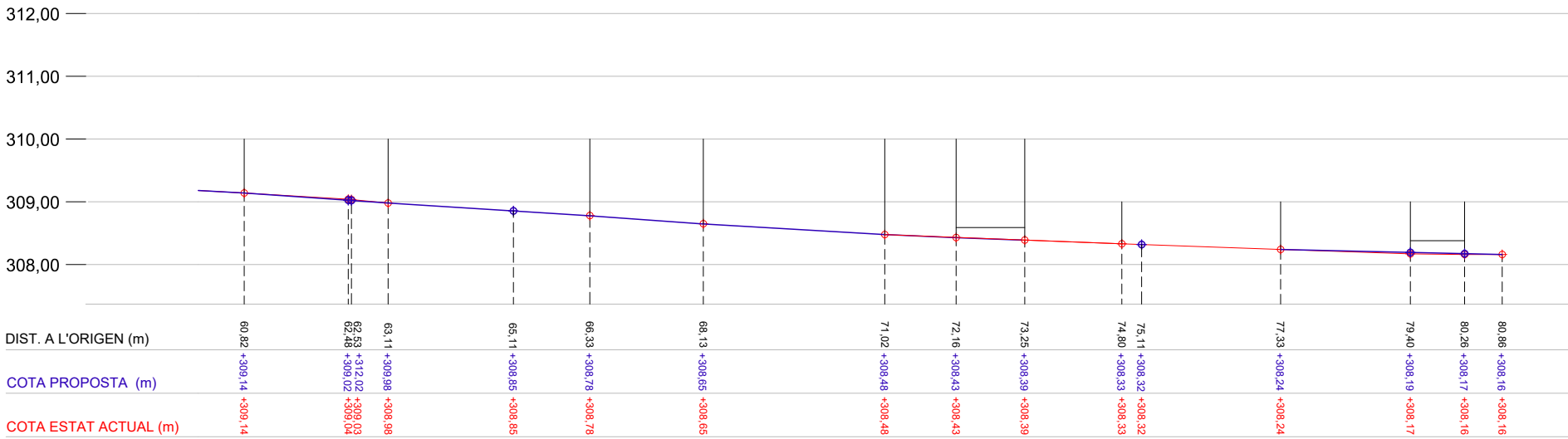
ALÇAT A1-A1' E1:100
