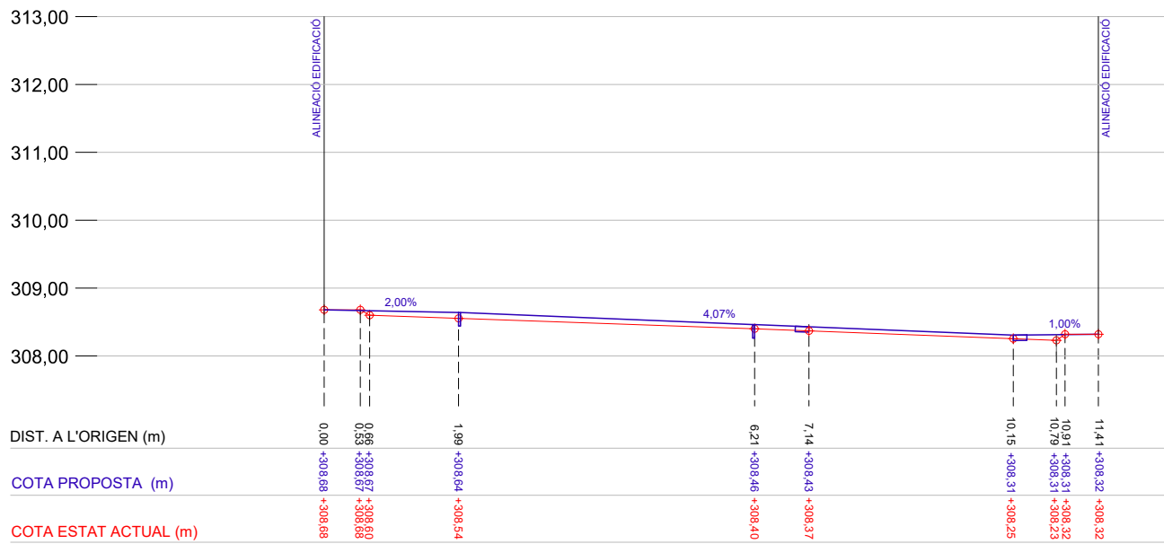
SECCIÓ 1 - CARRER CALVARI - D1 E1:100
