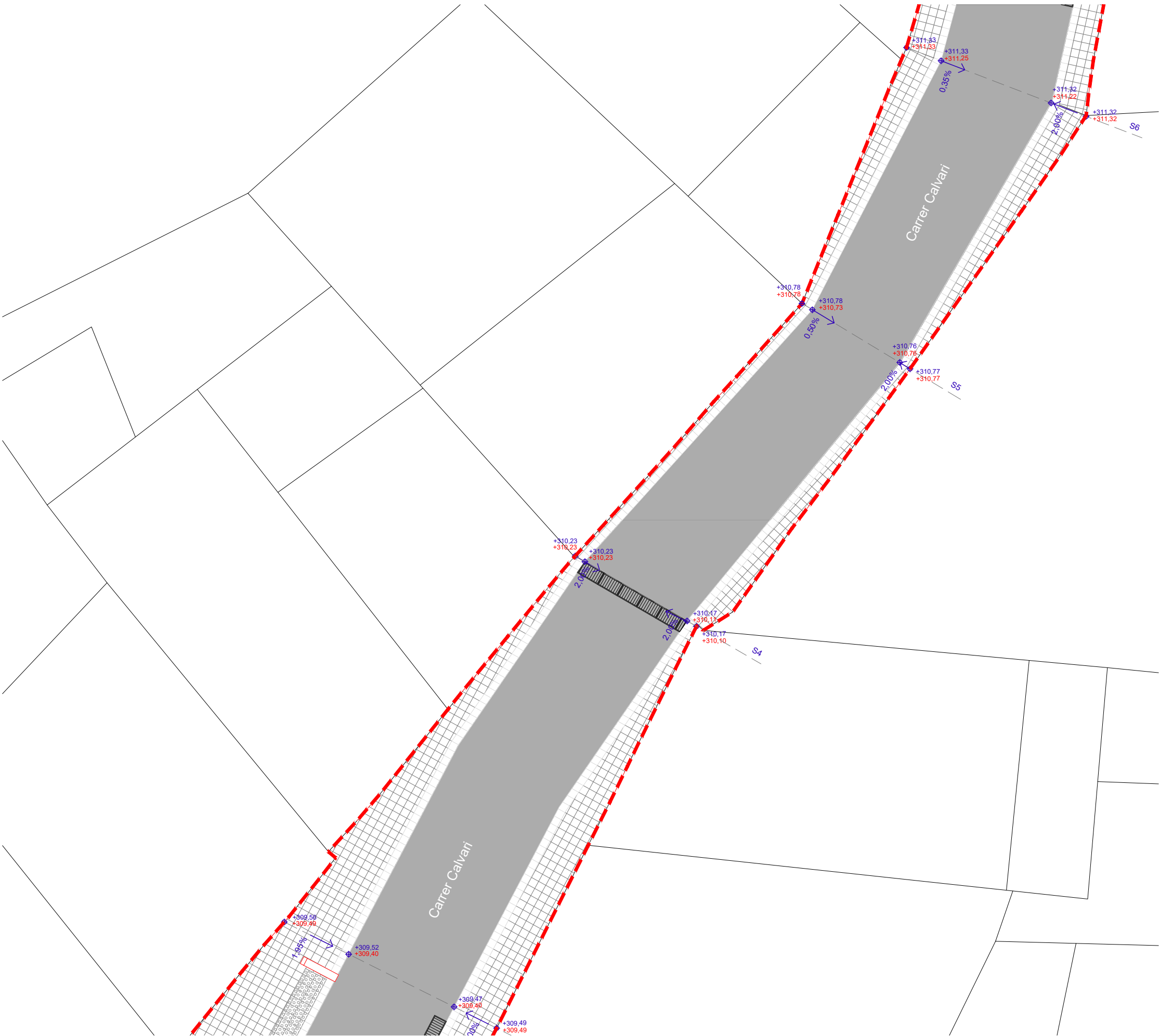
PLANTA PROPOSTA - CARRER CALVARI - D2 E1:100 - - - Àmbit d'Actuació
