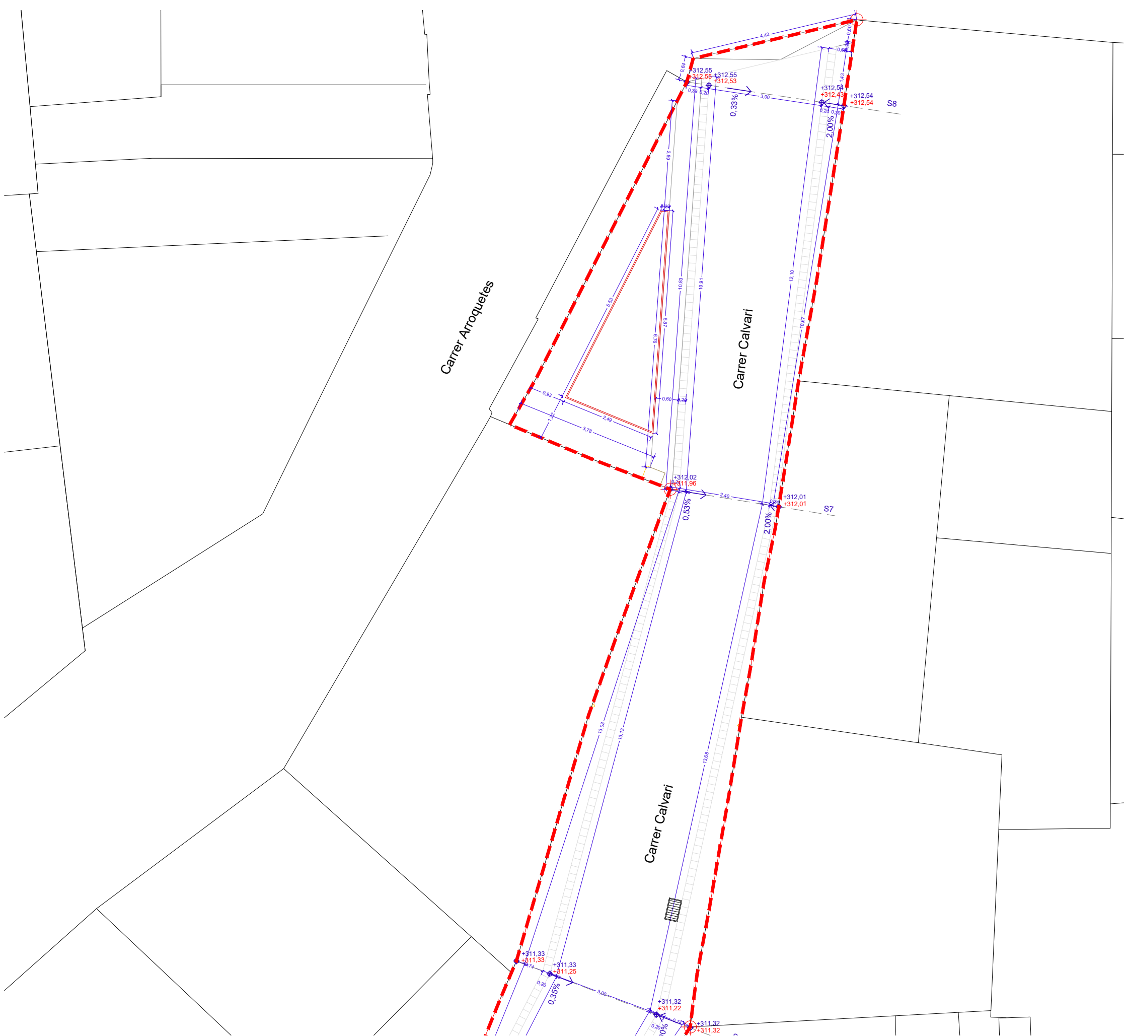
REPLANTEIG PROPOSTA - CARRER CALVARI - D3 E1:100
