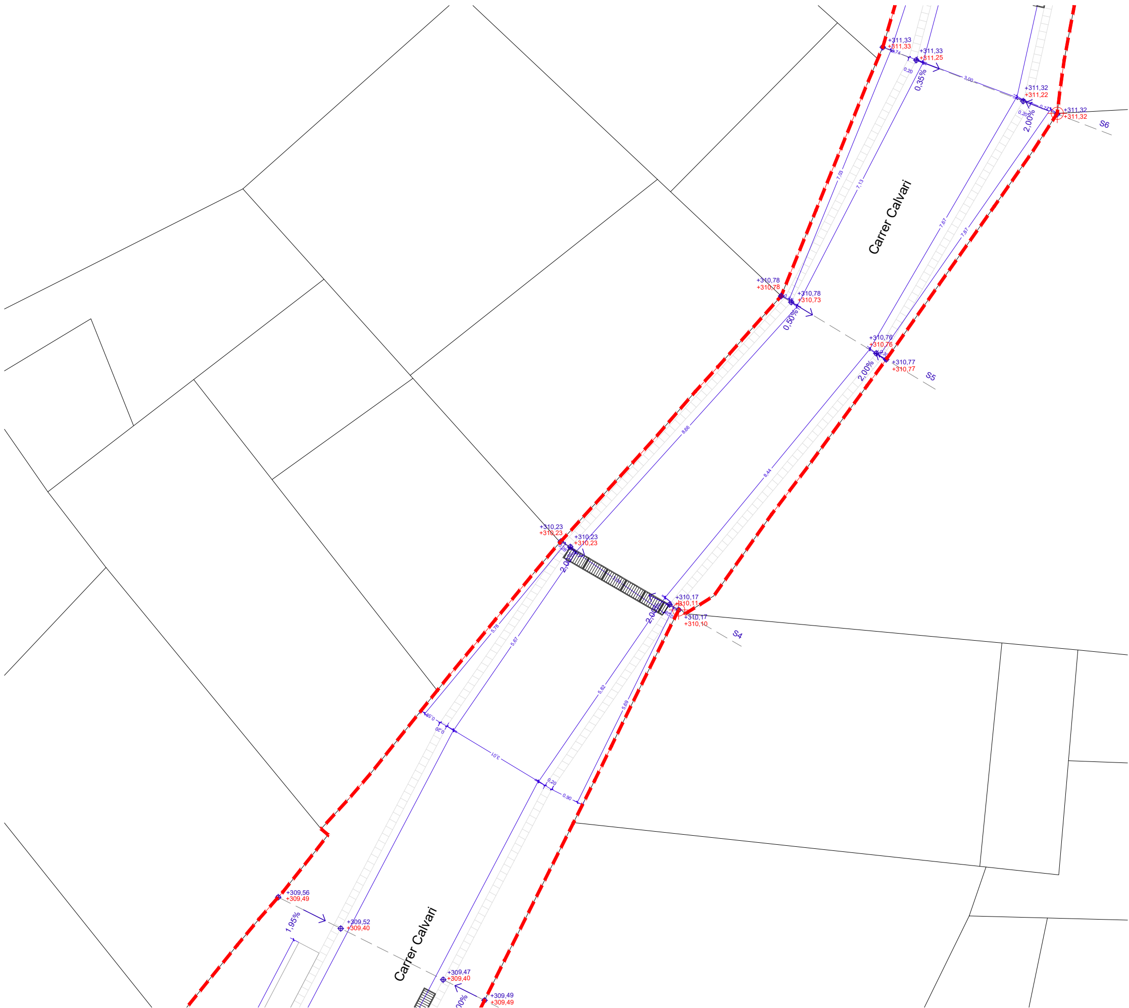
REPLANTEIG PROPOSTA - CARRER CALVARI - D2 E1:100
