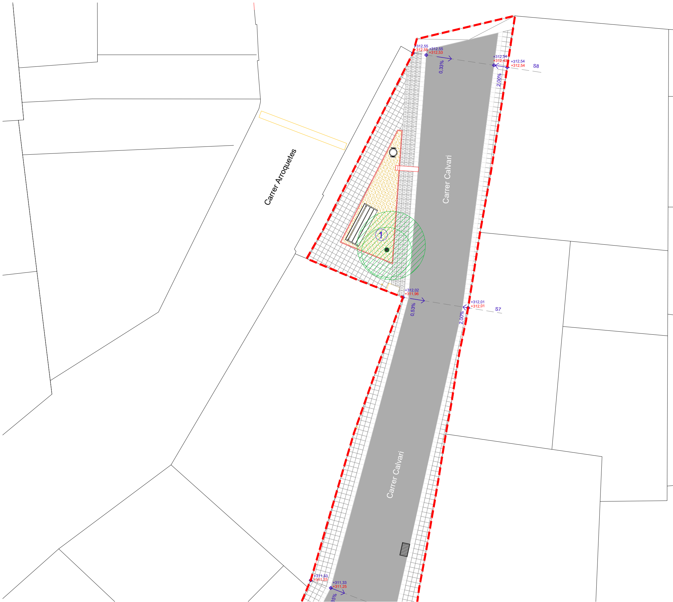
PLANTA PROPOSTA - CARRER CALVARI - D3 E1:100 - - - Àmbit d'Actuació
