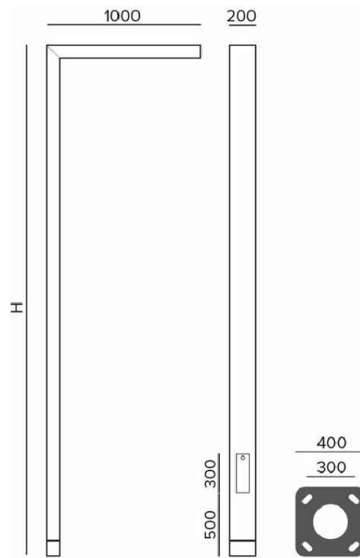
DETALL COLUMNA ENLLUMENAT MODEL TOMSK DE BENITOLIGHT O SIMILAR
