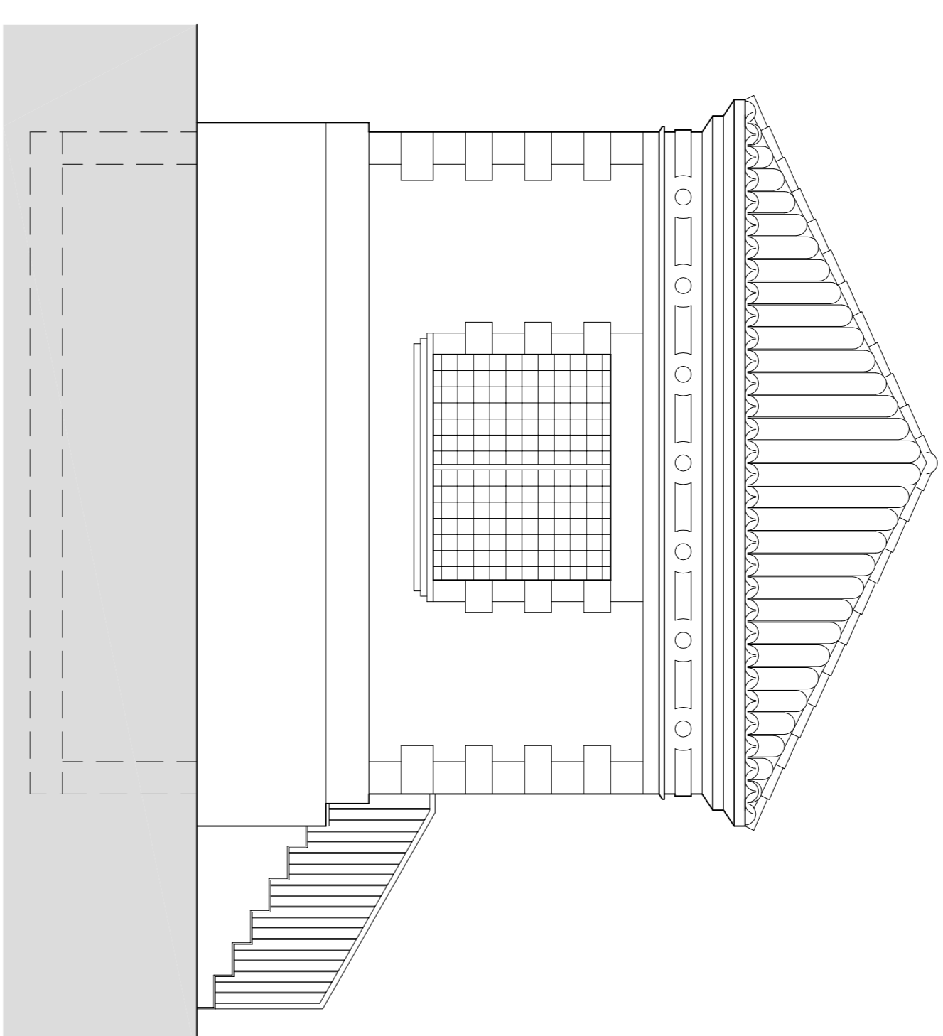
ALÇAT LATERAL NORD-EST E:1:50
