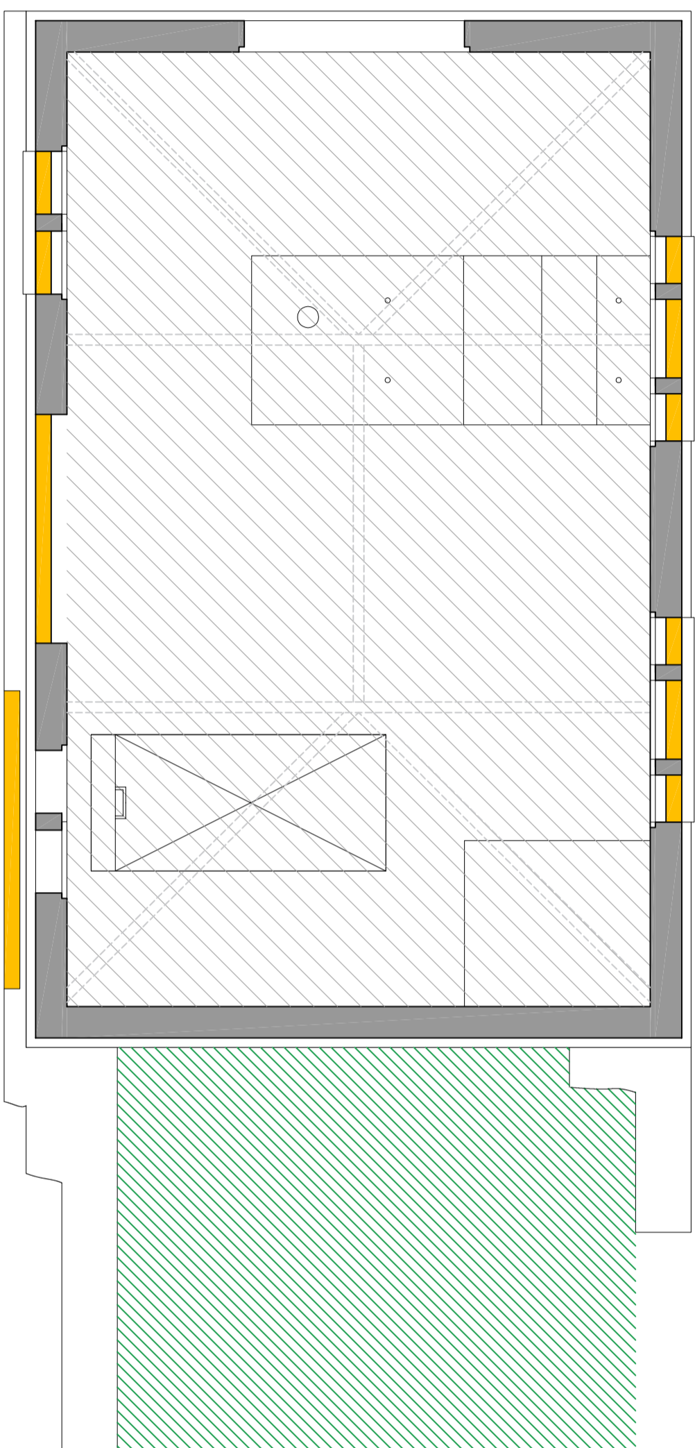
PLANTA SOTERRANI - ESTAT ACTUAL I ACTUACIONS E1:50
