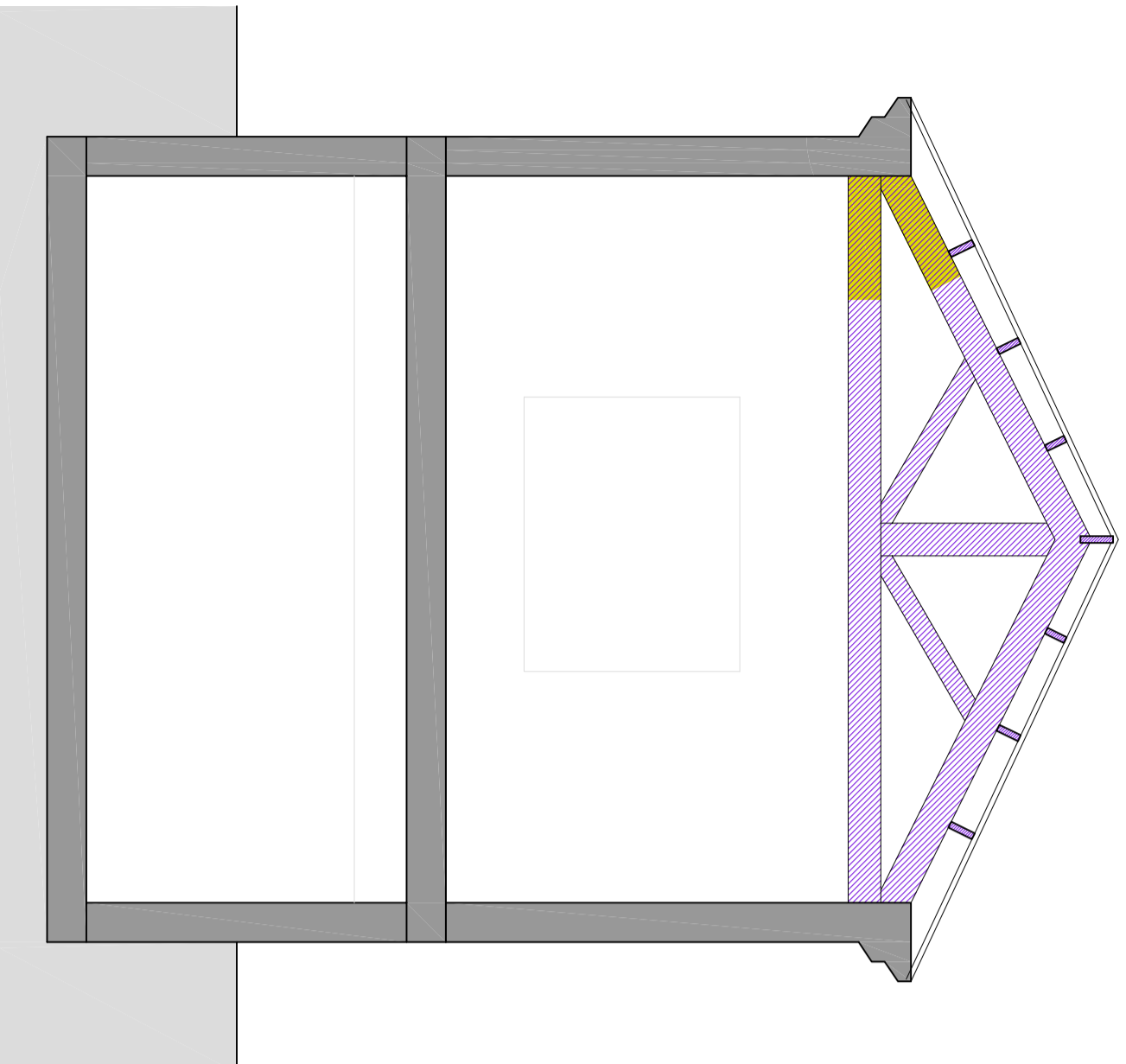
SECCIÓ TRANSVERSAL - ESTAT ACTUAL I ACTUACIONS E 1:50
