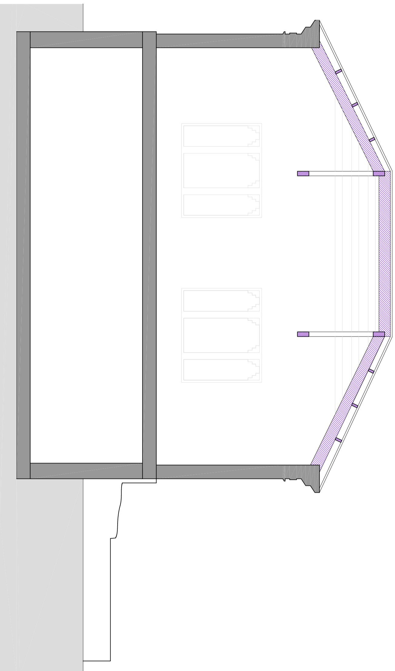
SECCIÓ LONGITUDINAL - ESTAT ACTUAL I ACTUACIONS E 1:50
