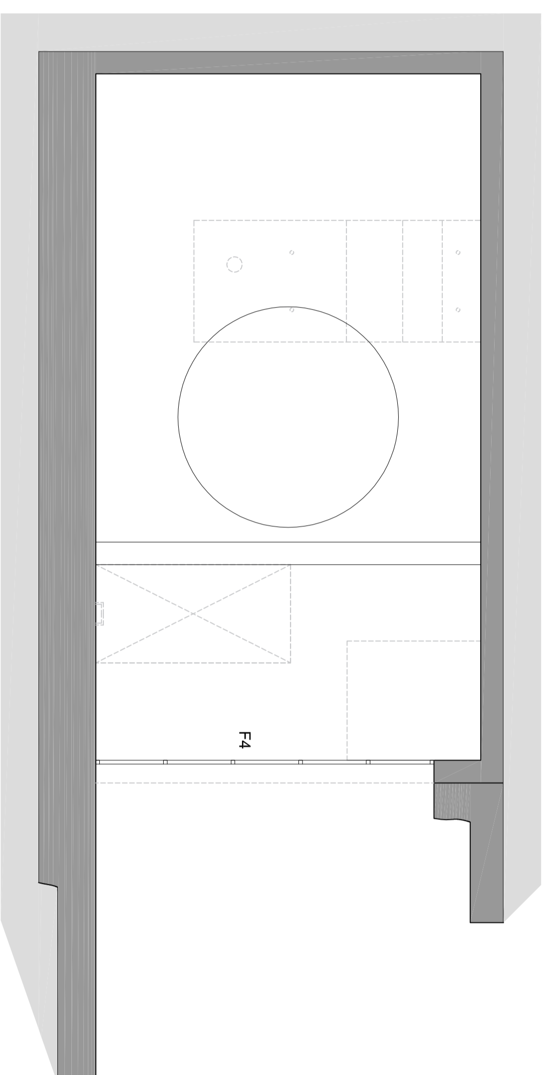
PLANTA SOTERRANI - PROPOSTA E1:50
